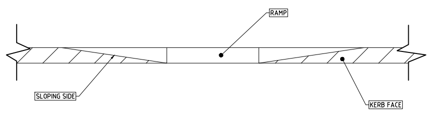
ELEVATION N.T.S
