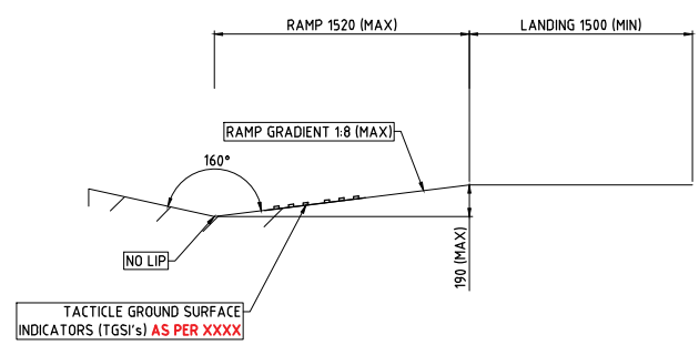
SECTION N.T.S
