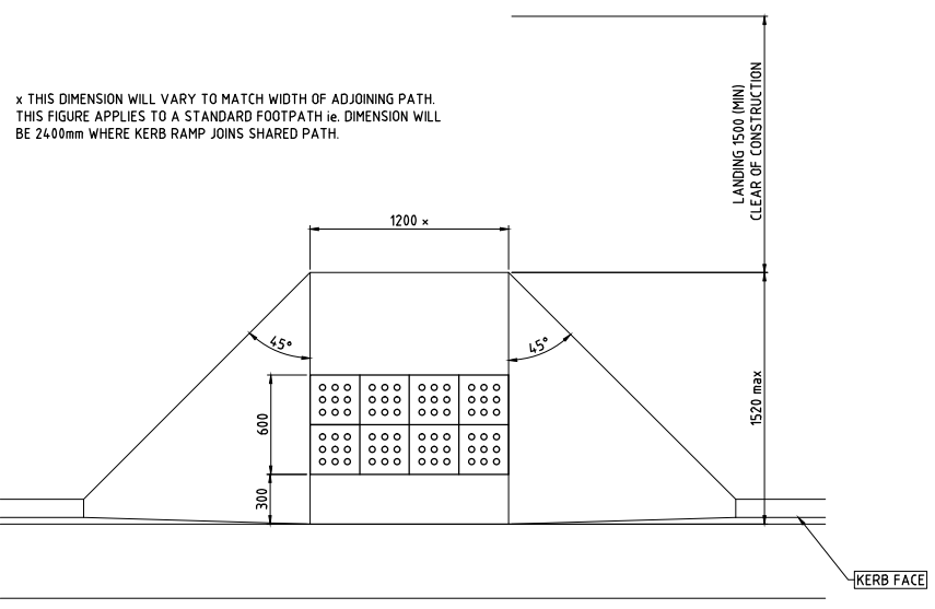
PLAN N.T.S
